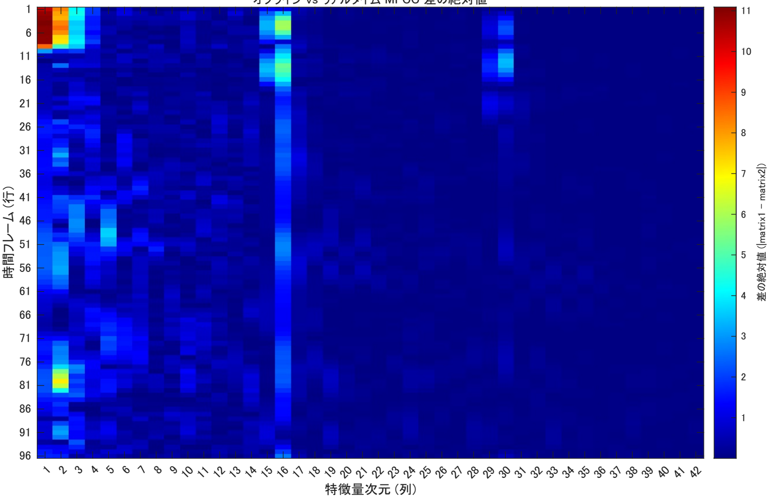
オフライン vs リアルタイム MFCC 差の絶対値
